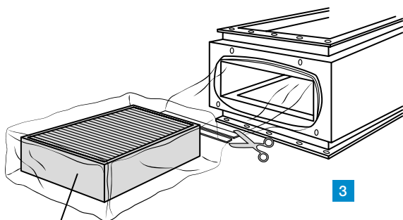
Oude filter
