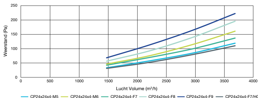
CP SERIE 96 MM
