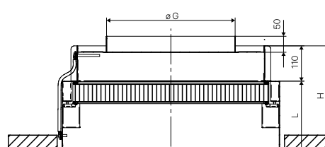
HL-HD-T Aansluiting bovenkant
