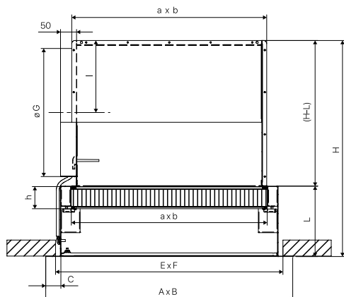
HL-HD-S Connexion latérale
